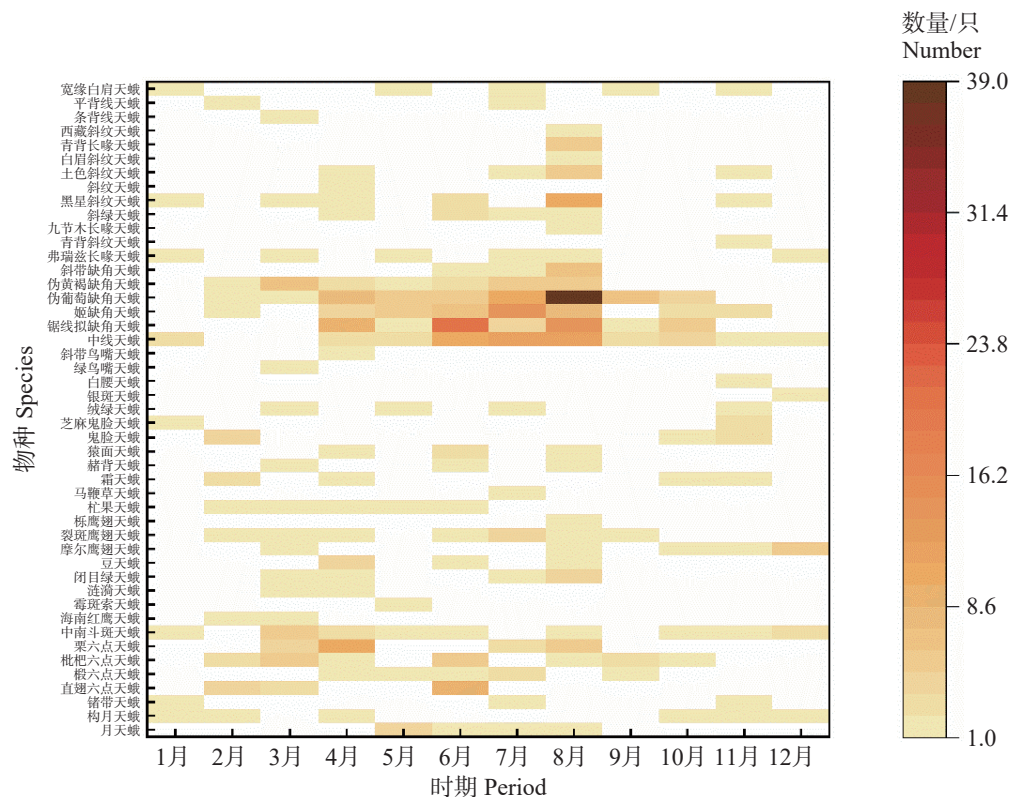
图4 黎母山景区天蛾科昆虫不同物种的飞行期分布与数量 Fig. 4 Flight period distribution and abundance of Sphingidae in Limu Mountain scenic area
