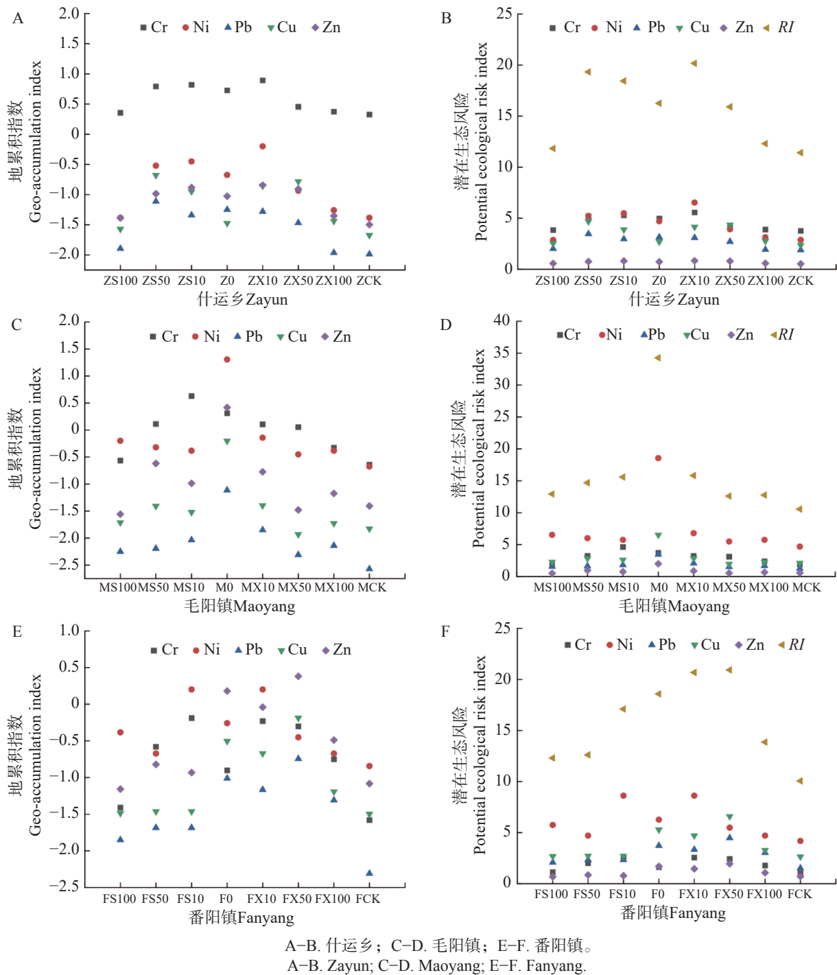
图2 土壤重金属的地累积指数和潜在生态风险指数
