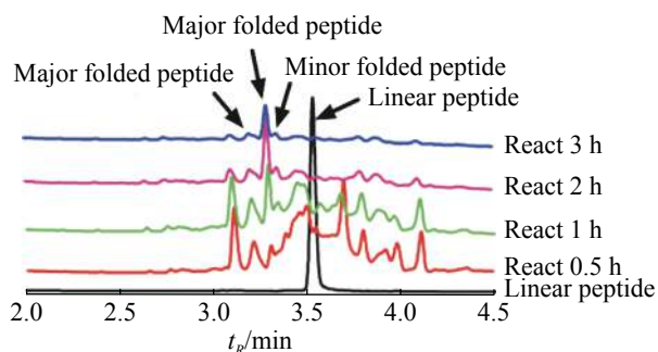
图 3 芋螺毒素 Lv68 氧化折叠反应的动态液相图
